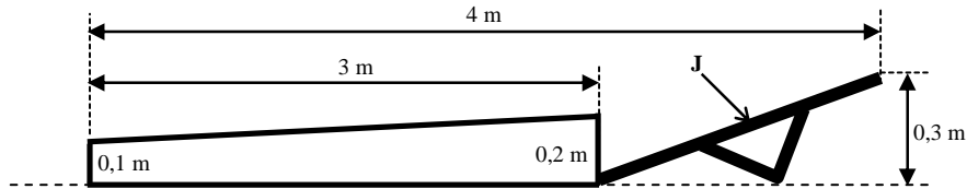
Der Rahmen von der Seite
